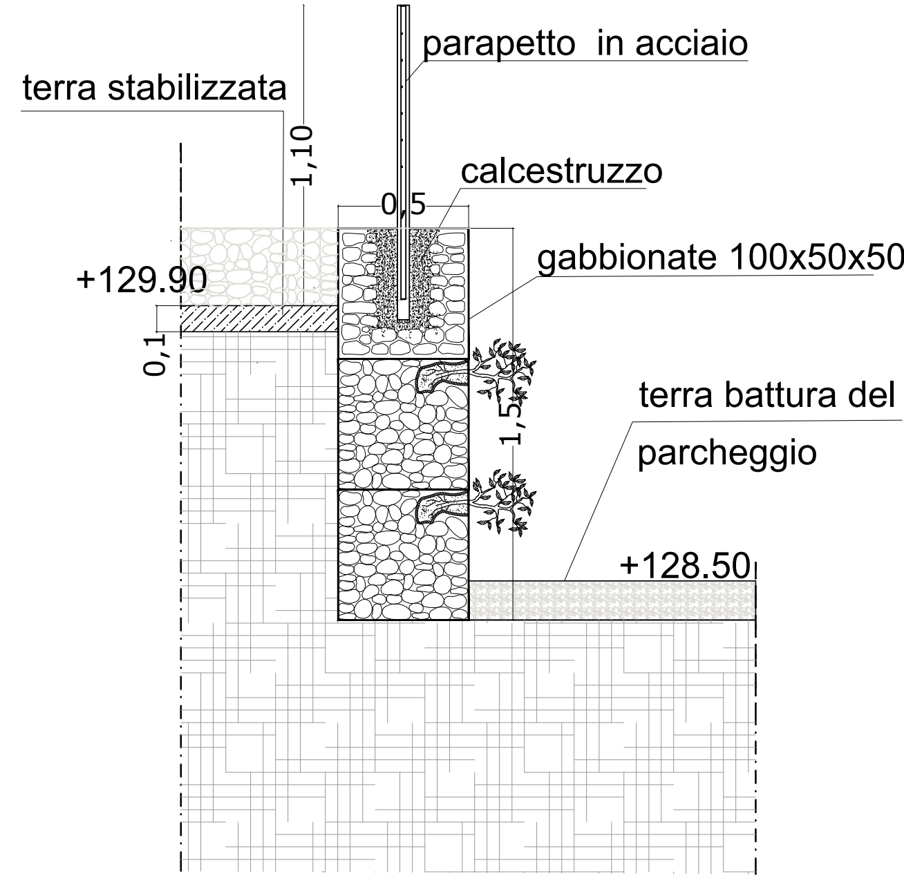
PARTICOLARE BALAUSTR (scala 1:200)
